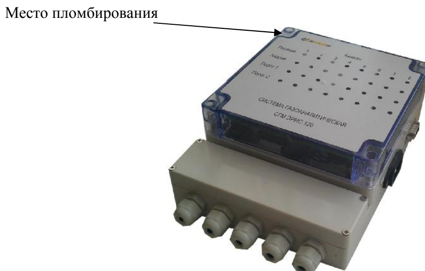
Рис. 3 Система газоаналитическая многофункциональная СГМ ЭРИС-120 (настенный BOX-11-13)
